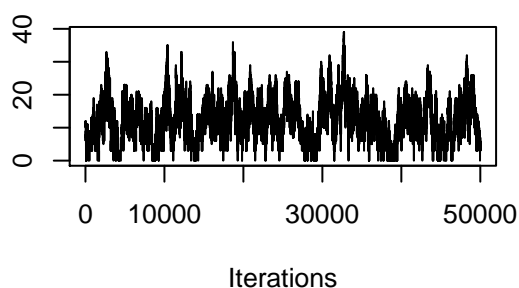
Trace of gwesp.fixed.0
