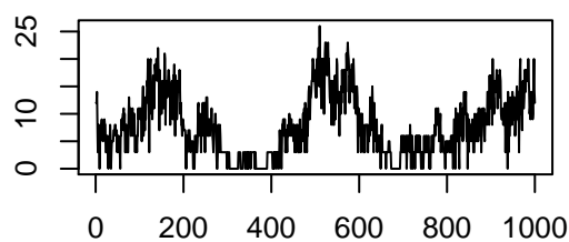
Trace of gwesp.fixed.0
